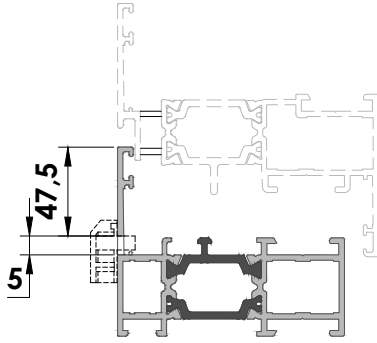
SECTION A-A Kesit A-A
